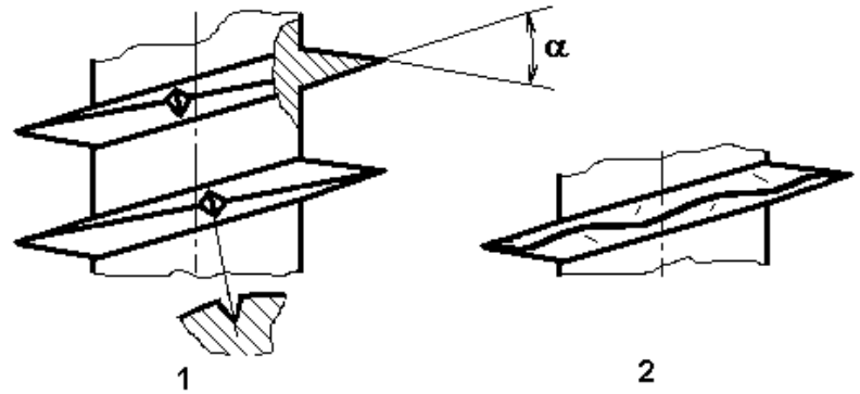
Для повышения самонарезающих свойств резьб можно уменьшить угол при вершине профиля резьбы \alpha , нарезать на резьбе специальную насечку (1), изготовить нитку резьбы с волнообразным профилем (2).
